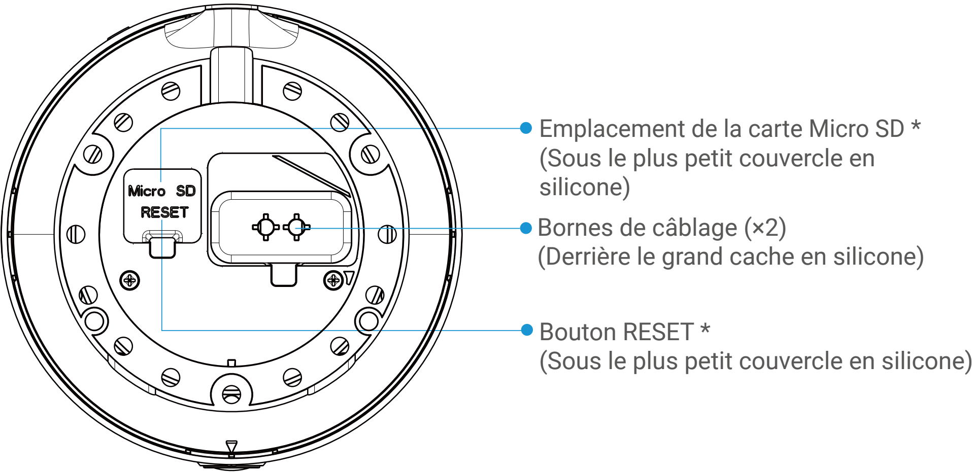
Vue inférieure
